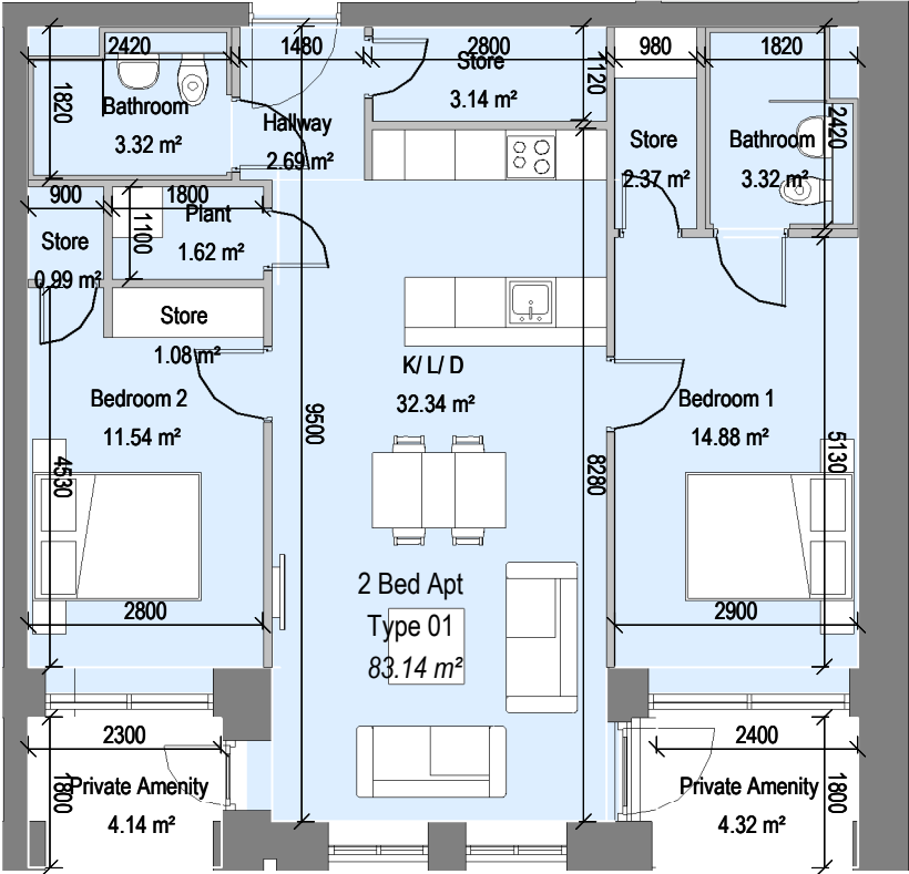
1 2 Bed Apt - Type 01 1 : 100
