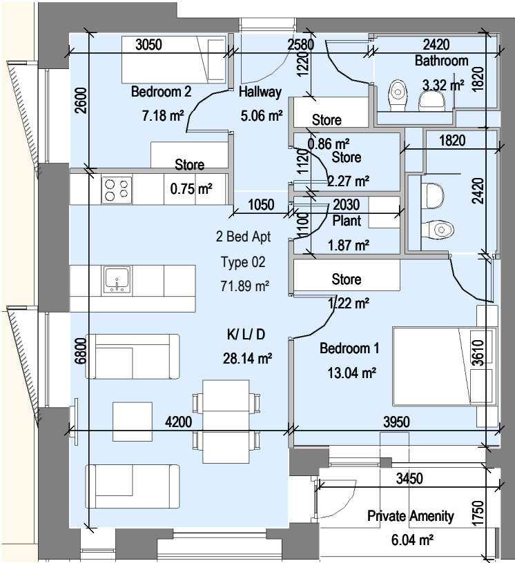
1 2 Bed Apt - Type 02 1 : 100
