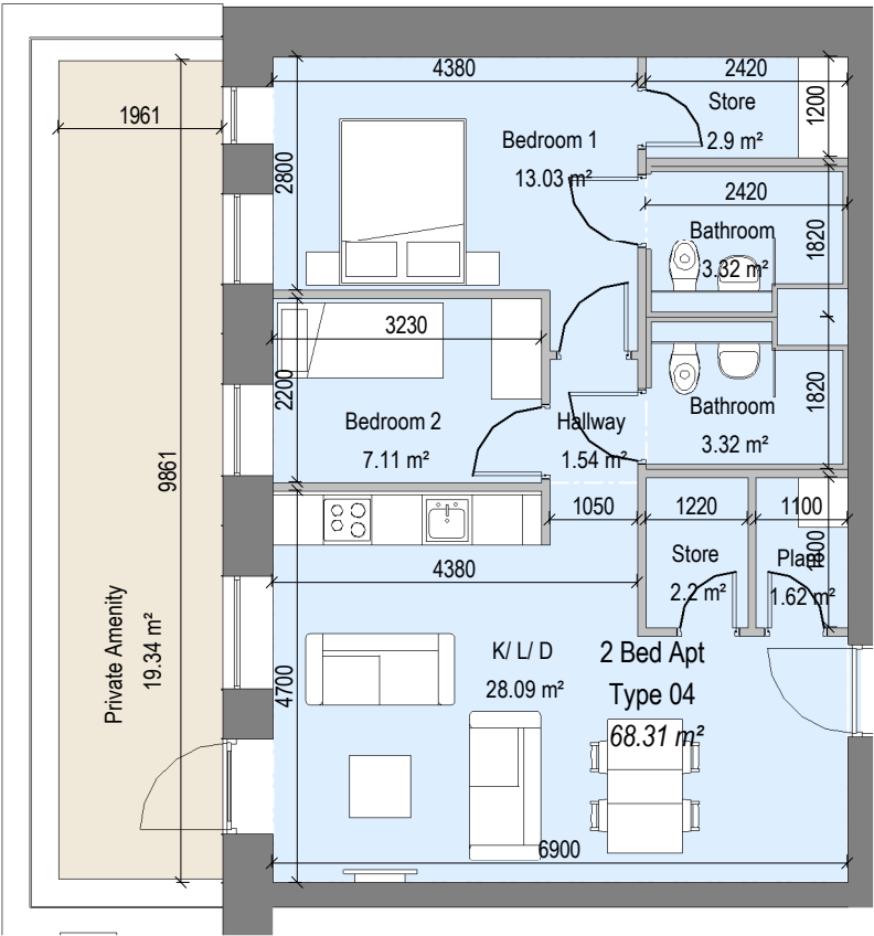
1 2 Bed Apt - Type 04 1 : 100
