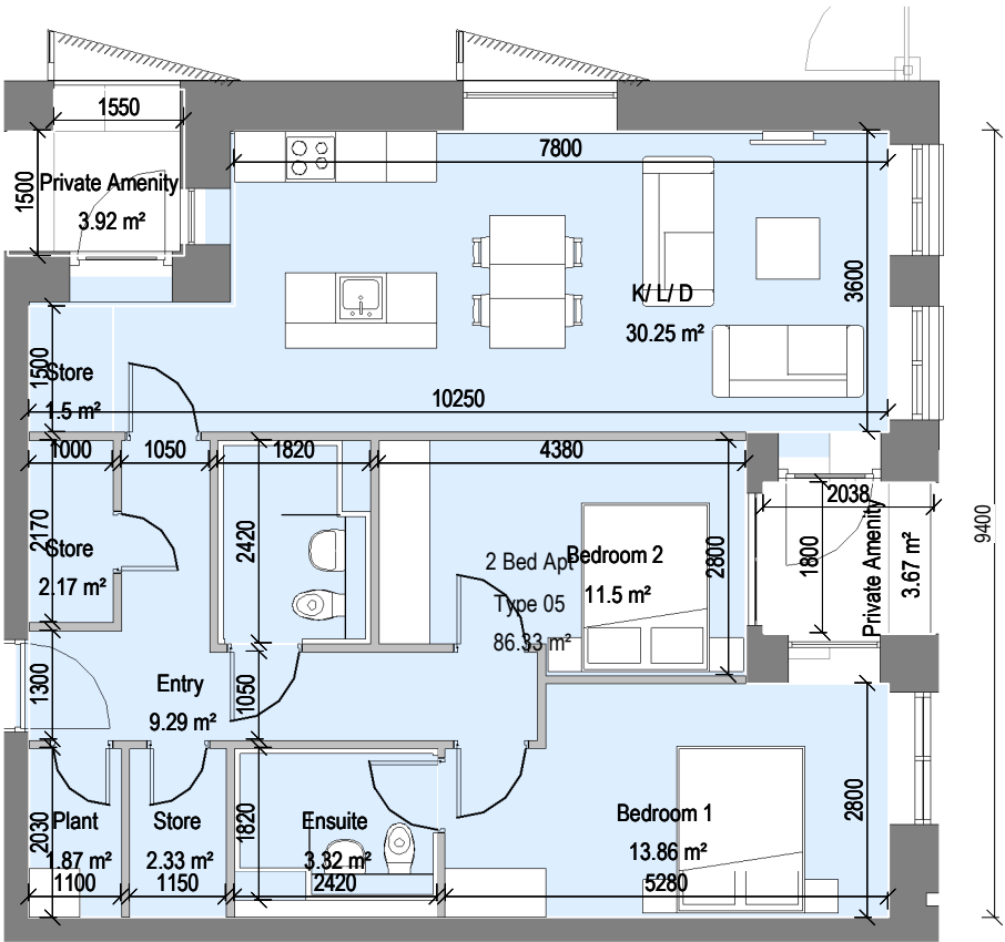
1 2 Bed Apt - Type 05 1 : 100
