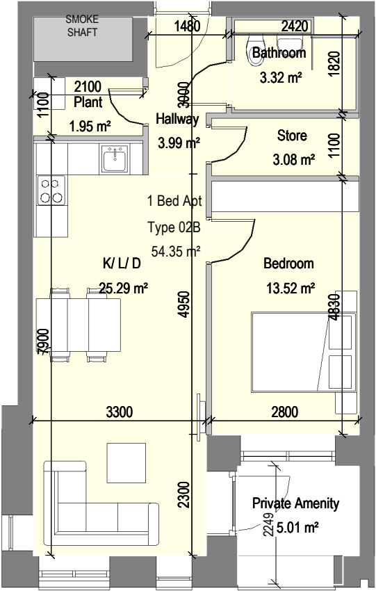
1 1 Bed Apt - Type 02B
