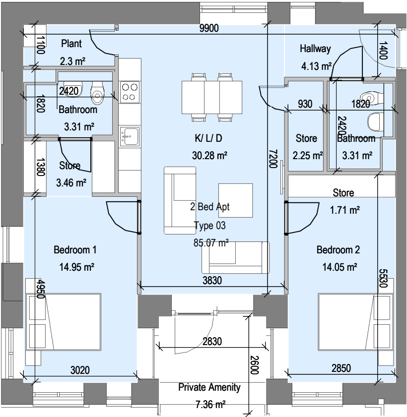
1 2 Bed Apt - Type 03 1 : 100
