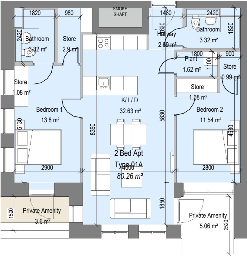
1 2 Bed Apt - Type 01A 1 : 100
