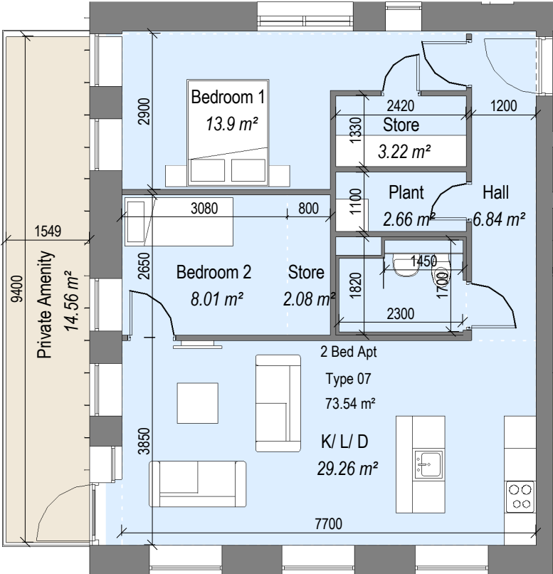
1 2 Bed Apt - Type 07 1 : 100
