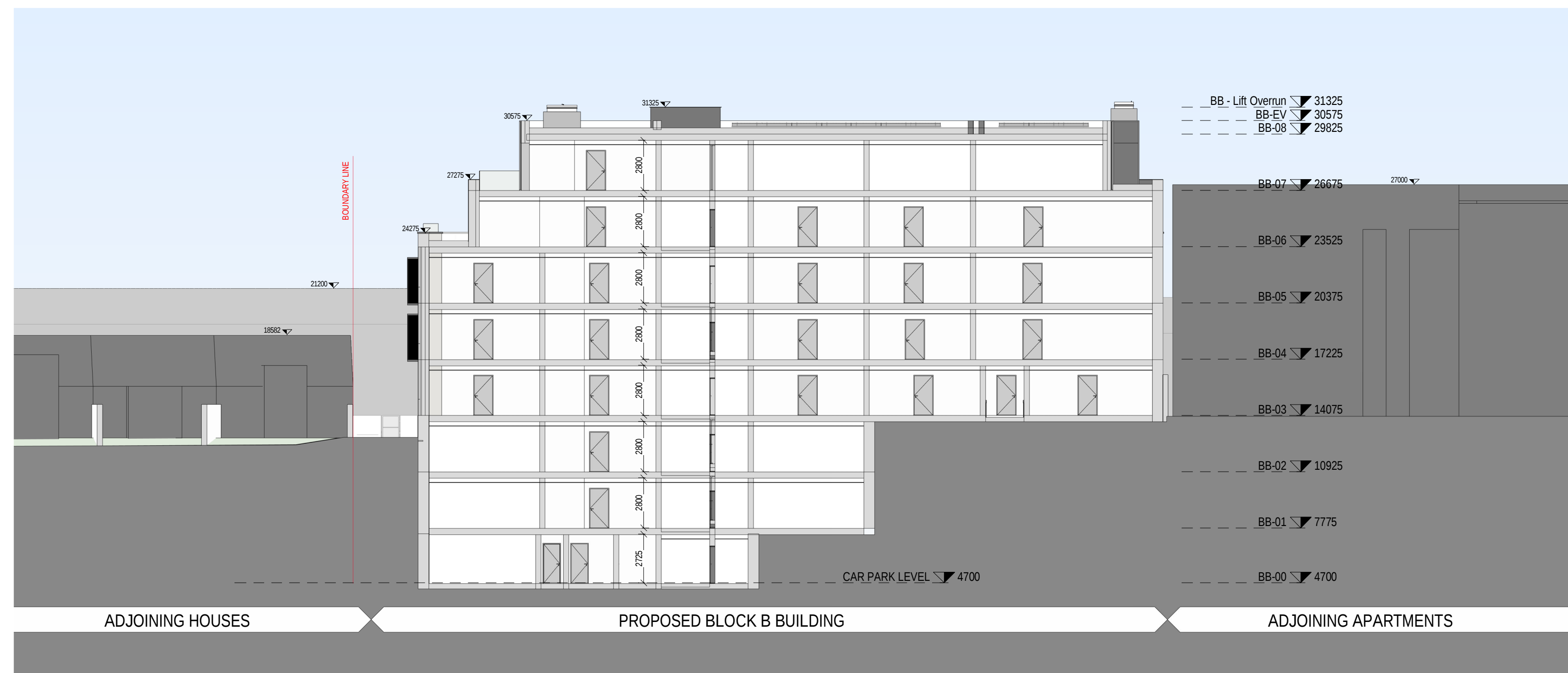
1 Section BB 1 : 200
